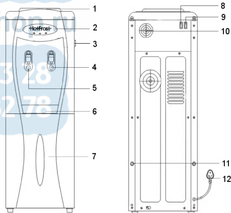
Рис.2 Схема аппарата V208XE...
